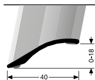
247 SK selbstklebend
