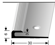
804 versenkt gebohrt
